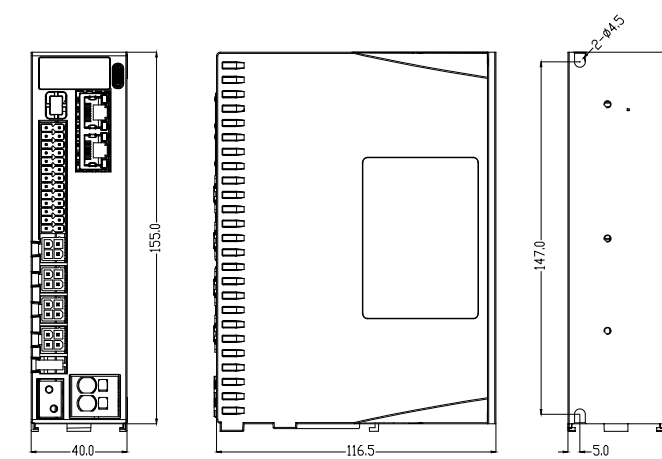
4DM3-EC安装尺寸图
