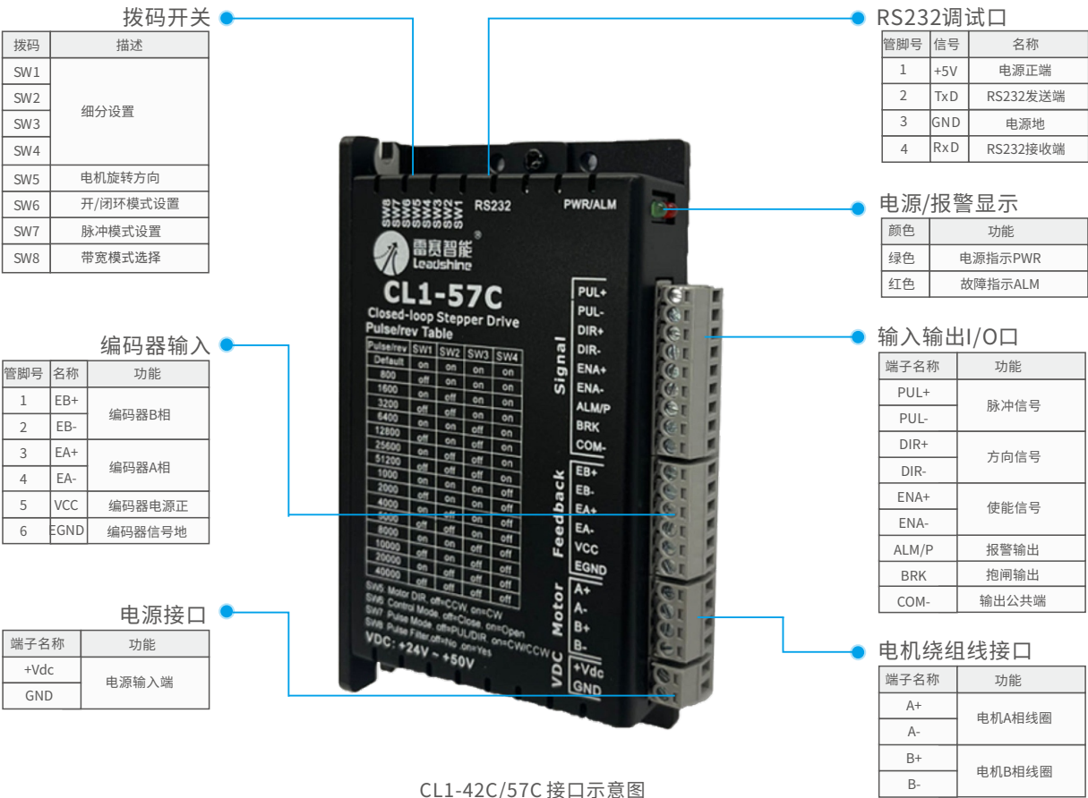
CL1-42C/57C 接口示意图
