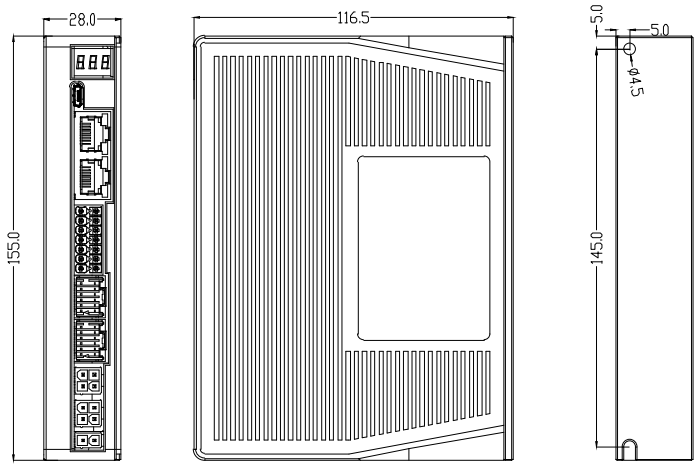
2CL3-EIP503/507安装尺寸图
