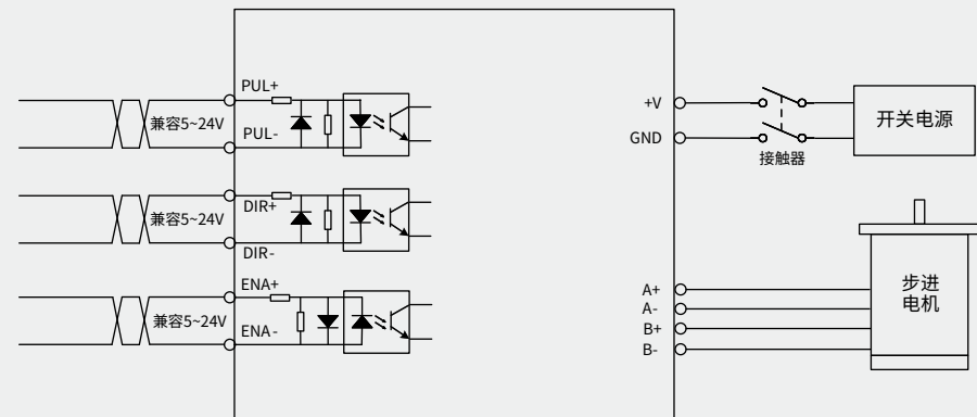
DM1-422C、DM1-432C、DM1-442C、DM1-542C、DM1-556C接线图
