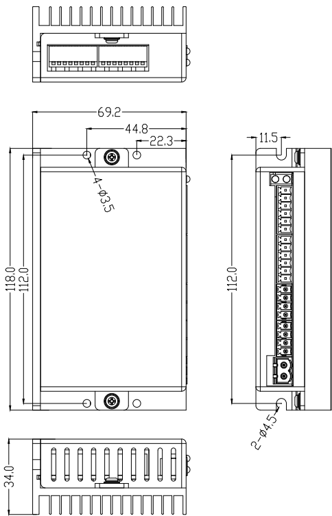
2DM57C 安装尺寸图
