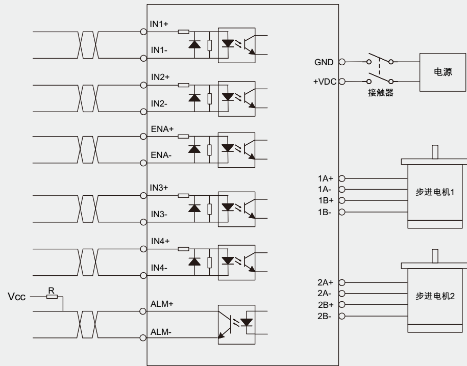
2DM57C-V、2DM86C-V电气接线图
