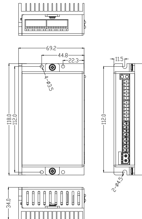
2DM57C-IO/-V/-A安装尺寸图
