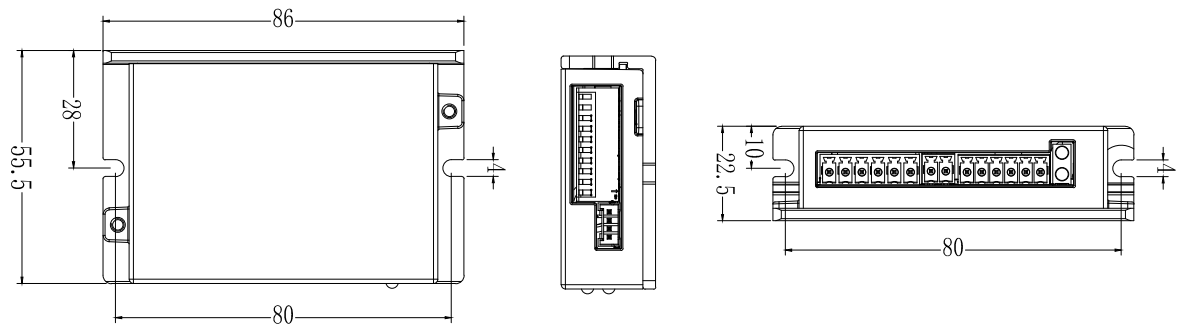
DM1-422、DM1-432安装尺寸图
