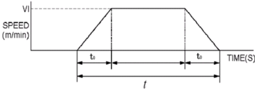
图3：运行曲线
