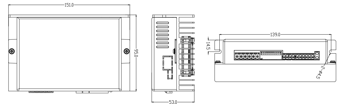
DM1-860C安装尺寸图
