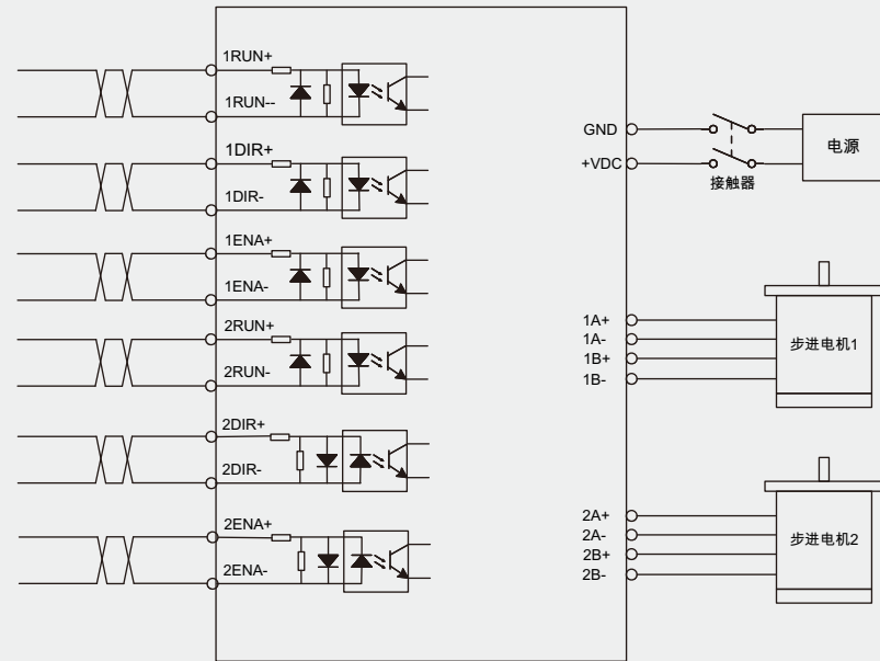
2DM57C-IO、2DM86C-IO电气接线图
