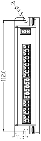
CL1-42C/57C安装尺寸图
