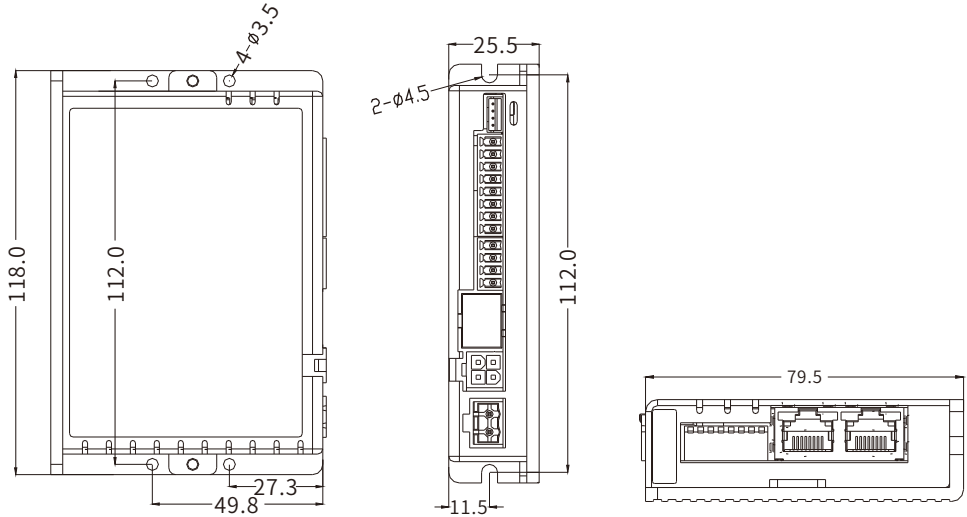
DM2B-RS522/542/556/570安装尺寸图
