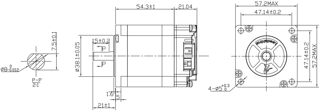
iCL57A-RS13
