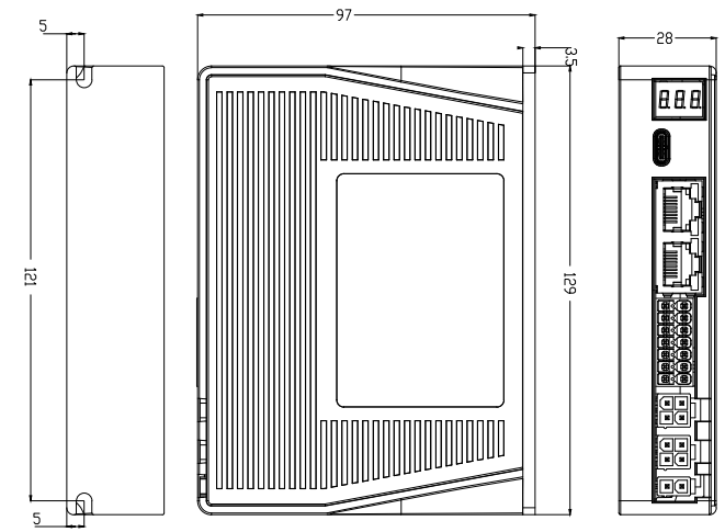
2DM3-EC432S安装尺寸图
