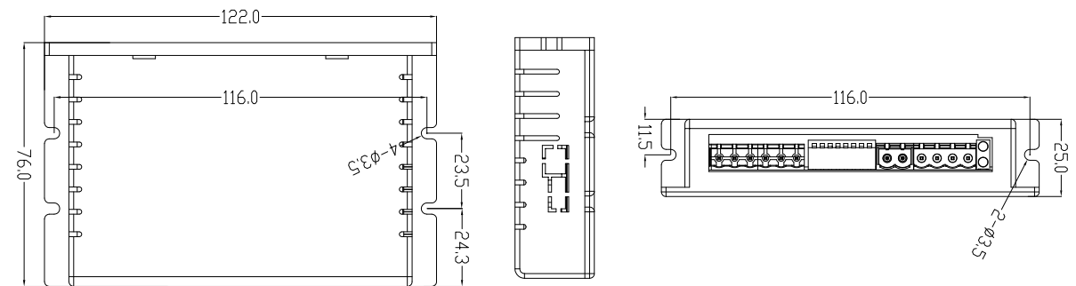
DM1-442C安装尺寸图
