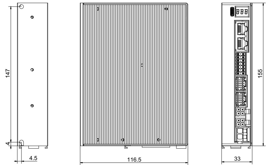
2CL3-EC808T安装尺寸图
