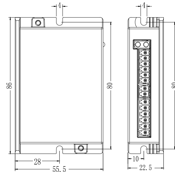
DM1-IO422C安装尺寸图
