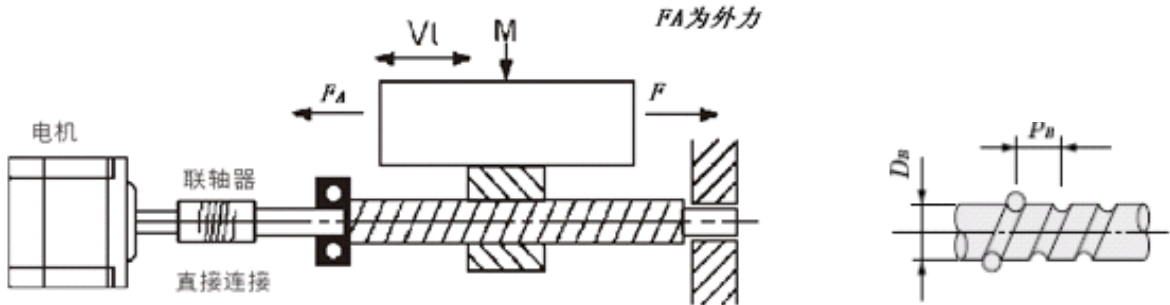
图1：丝杠水平运动
