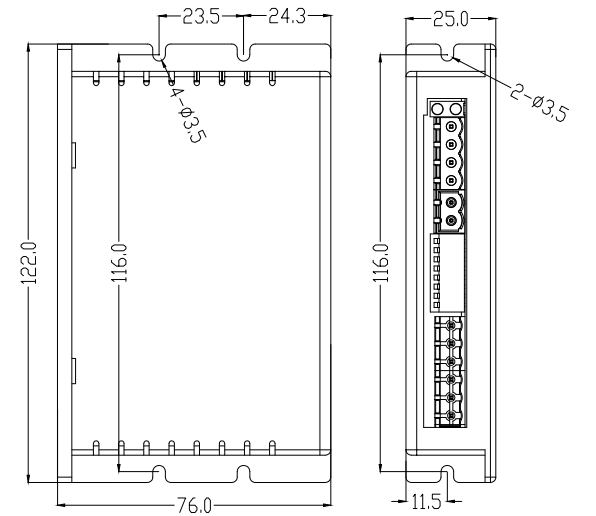
DM1-IO442C安装尺寸图
