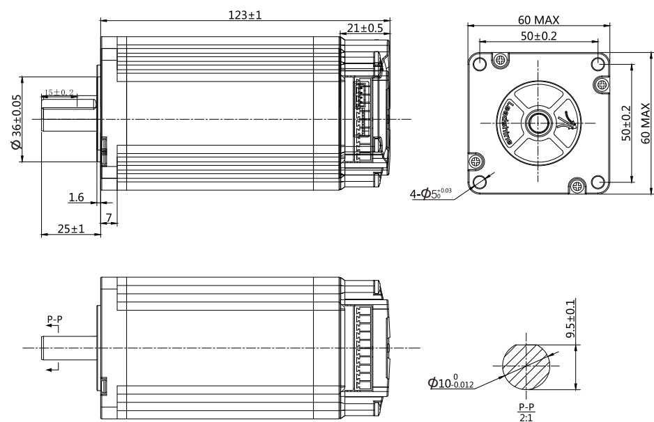
iCL60-35 (V2.0)
