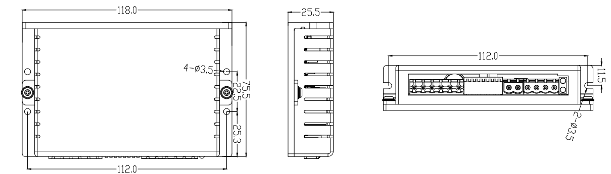
DM1-542C、DM1-556C安装尺寸图
