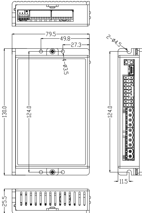
2DM57 安装尺寸图
