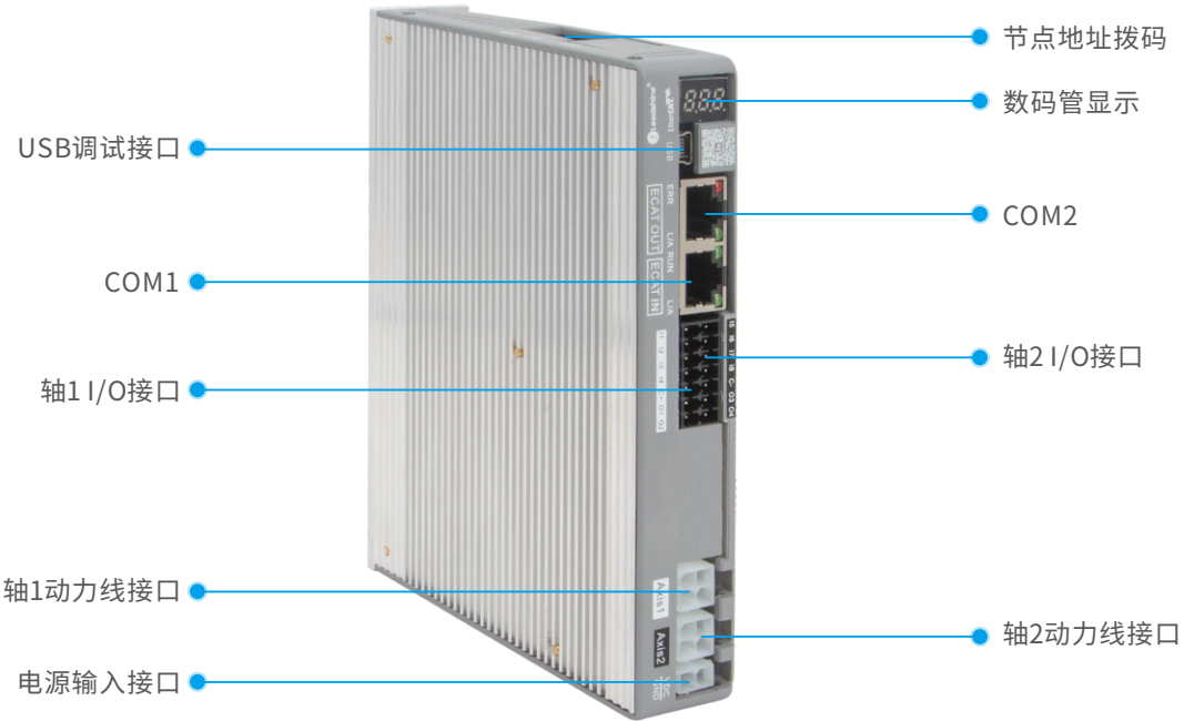
2DM3-EIP522/556/870接口说明
