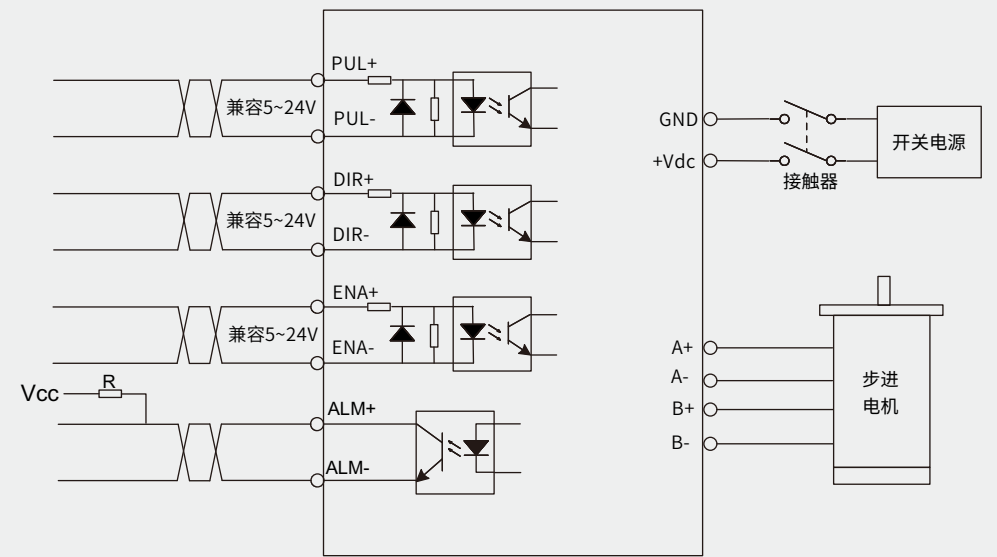
DM1-422、DM1-432接线图
