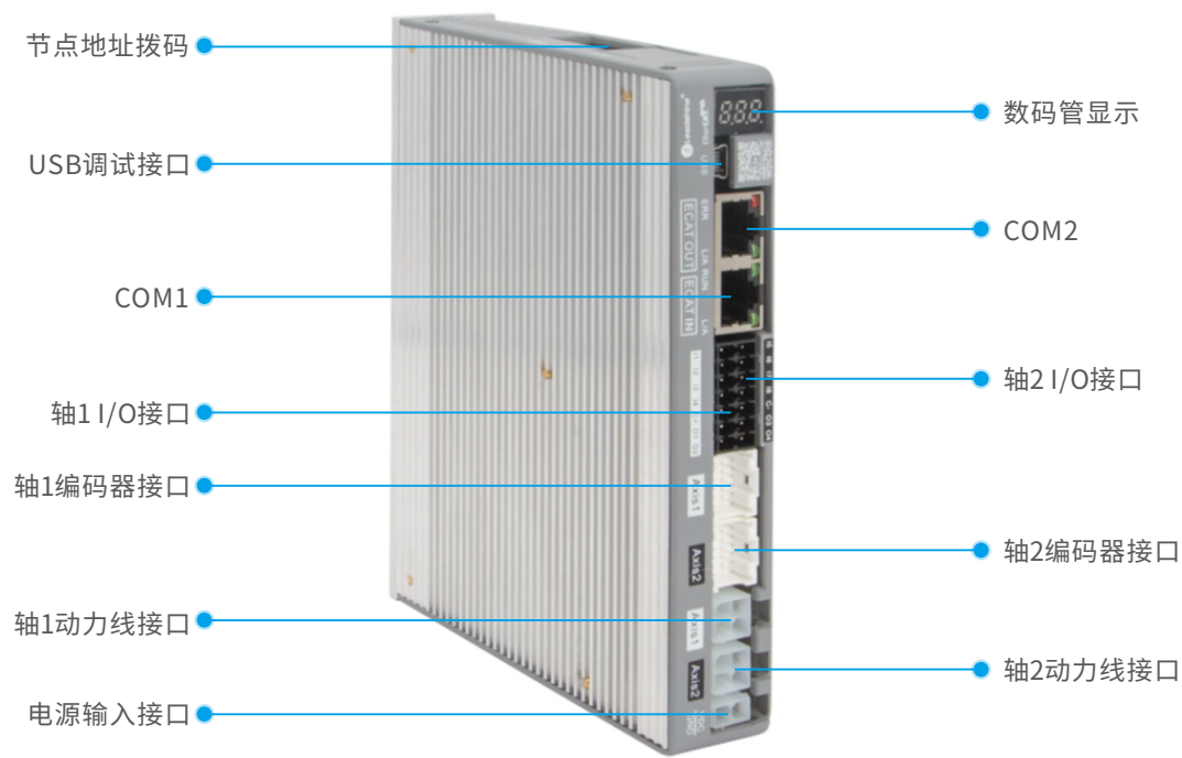
2CL3-EIP503/507接口示意图
