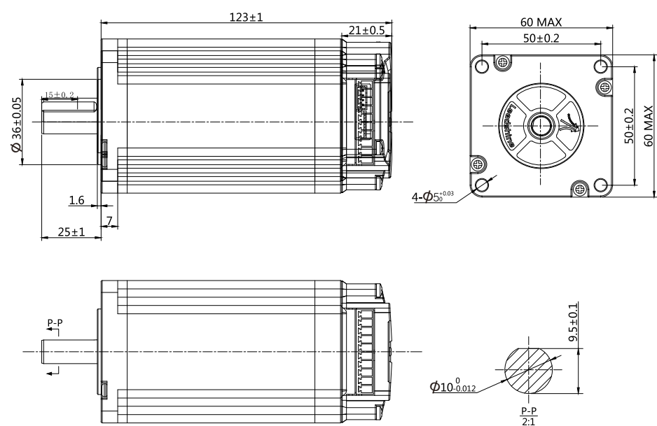
iDM60-35 (V2.0)
