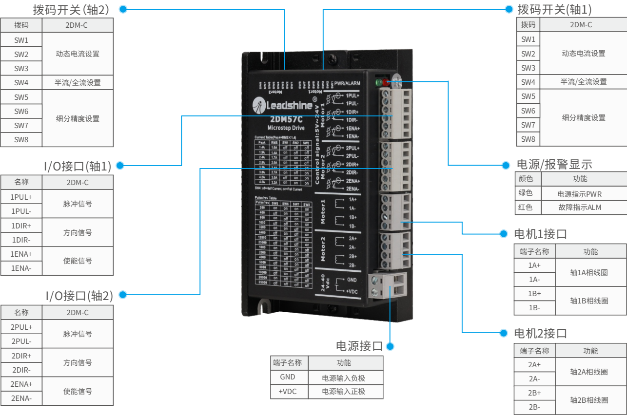
2DM57C (2DM42T) 接口说明
