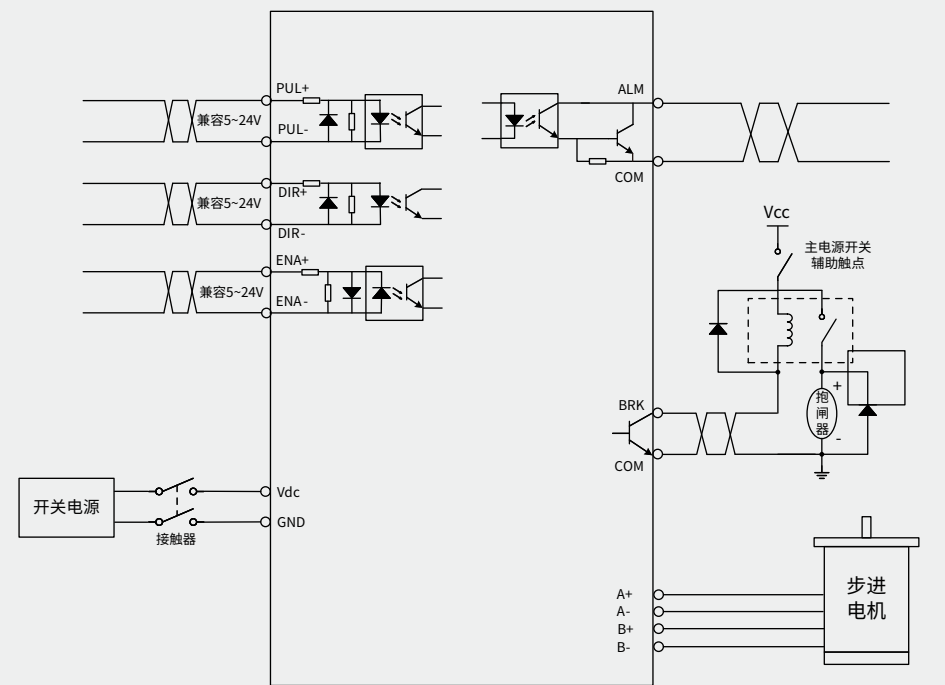
DM1-542、DM1-556、DM1-870接线图
