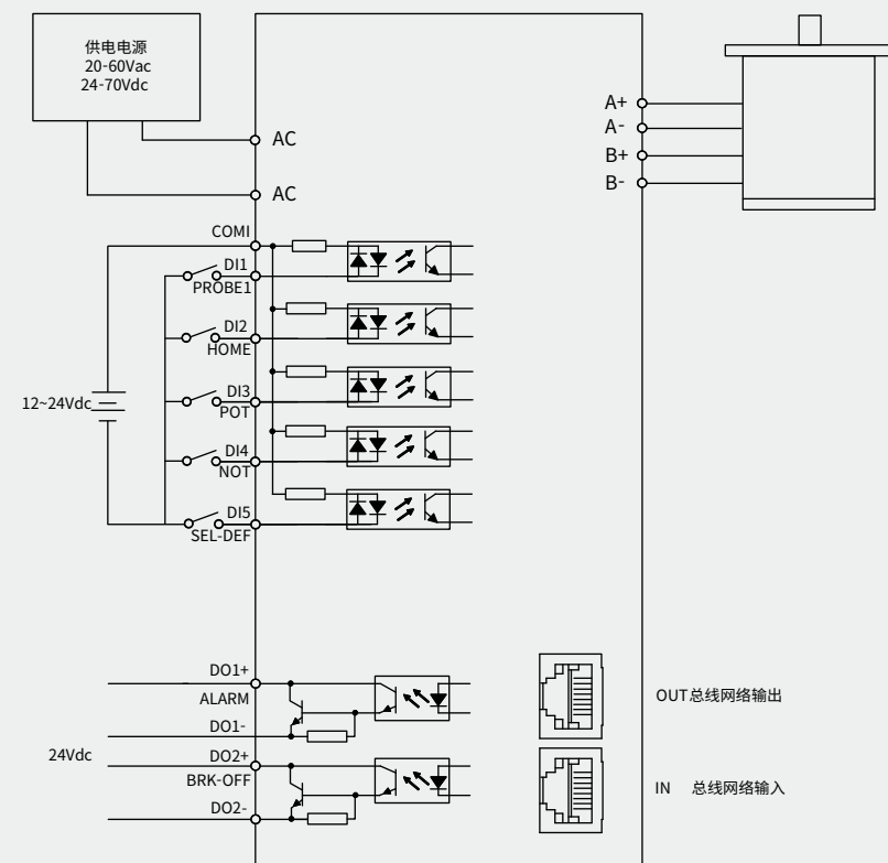
DM3B-EC882AC电气接线图
