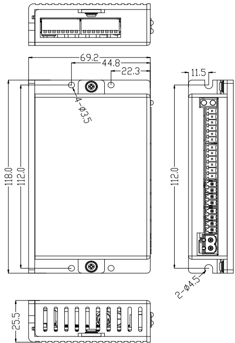
2DM42T 安装尺寸图
