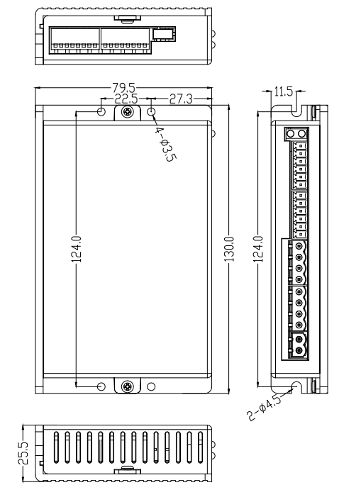
2DM86C-IO/-V/-A安装尺寸图
