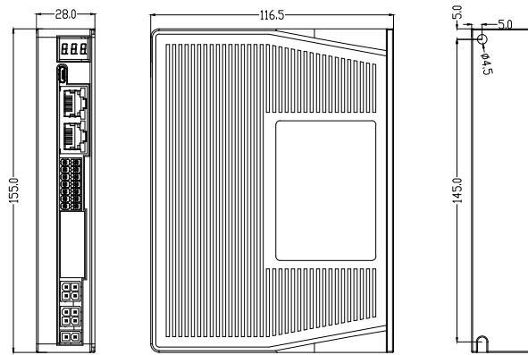
2DM3-EIP522/556/870安装尺寸图
