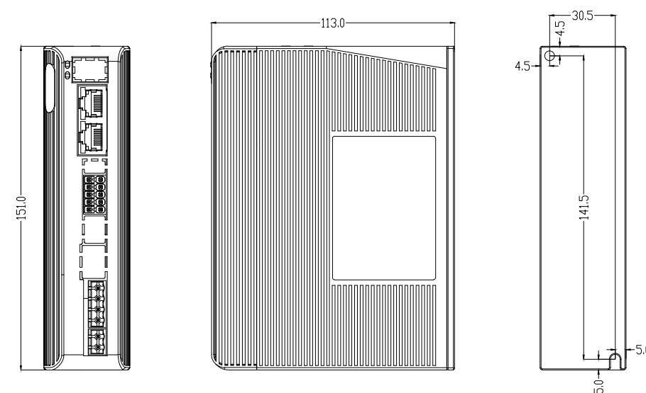
DM3B-EC882AC安装尺寸图
