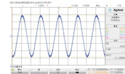
图6 57CM23电机在60rpm时的绕组电流波形
