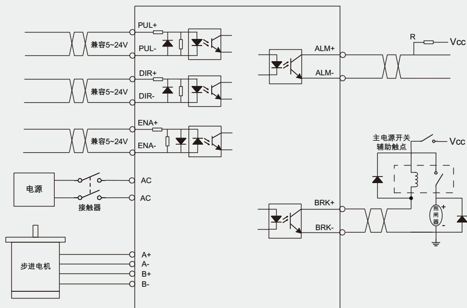
DM1-860C接线图
