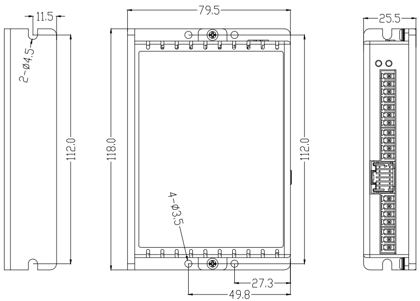
CL1-503/CL1-507安装尺寸图
