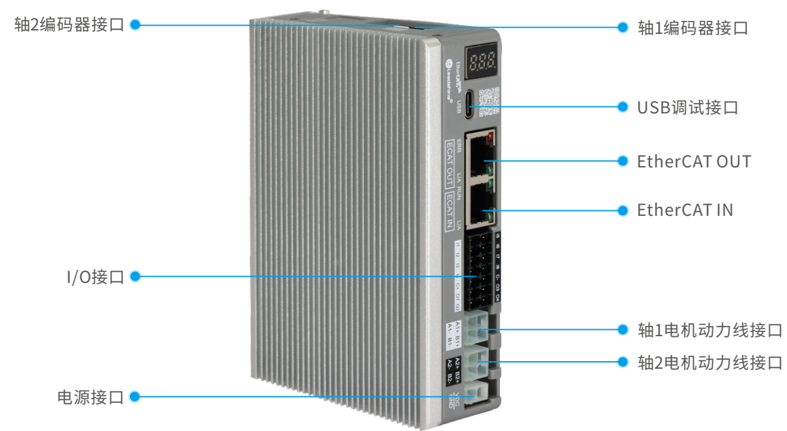
2CL3-EC507T/403T接口示意图
