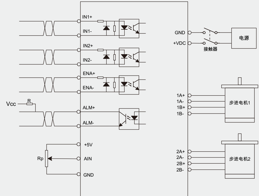
2DM57C-A、2DM86C-A电气接线图
