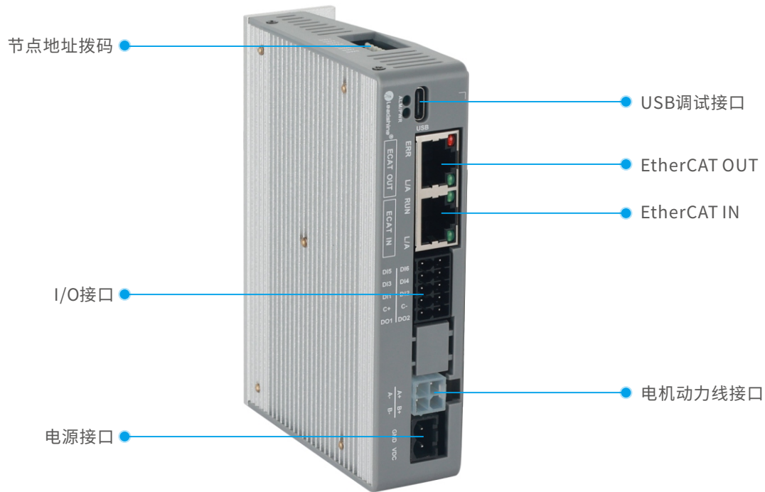
DM3B-EC522/542/556/570接口示意图
