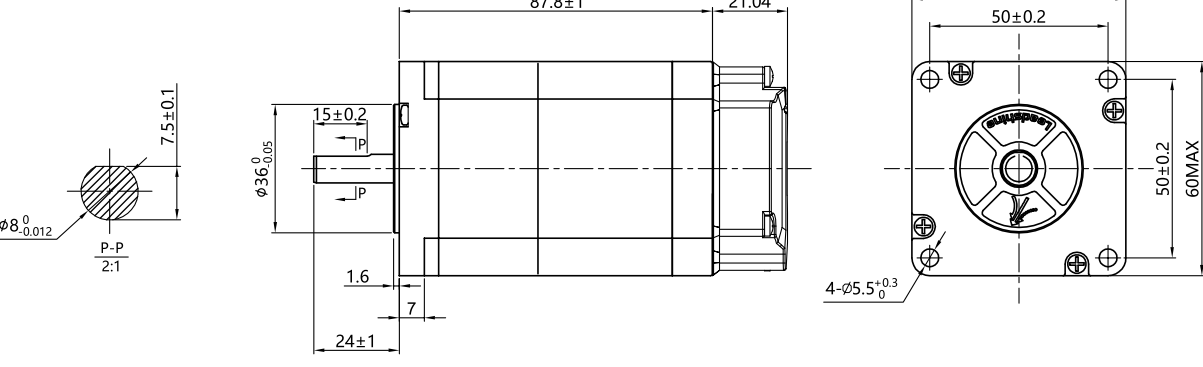
iCL60A-RS30
