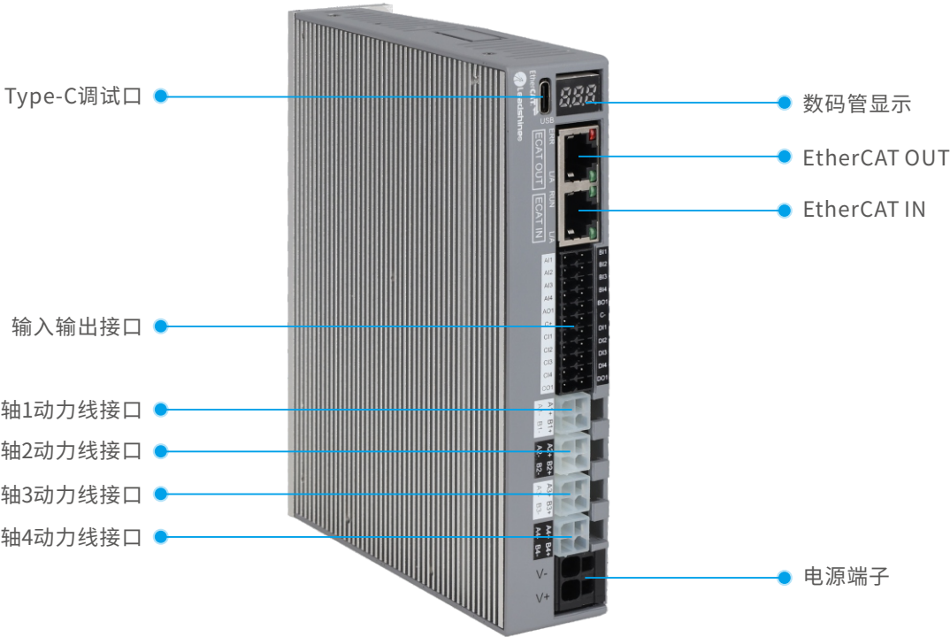
4DM3C-EC432/556接口说明
