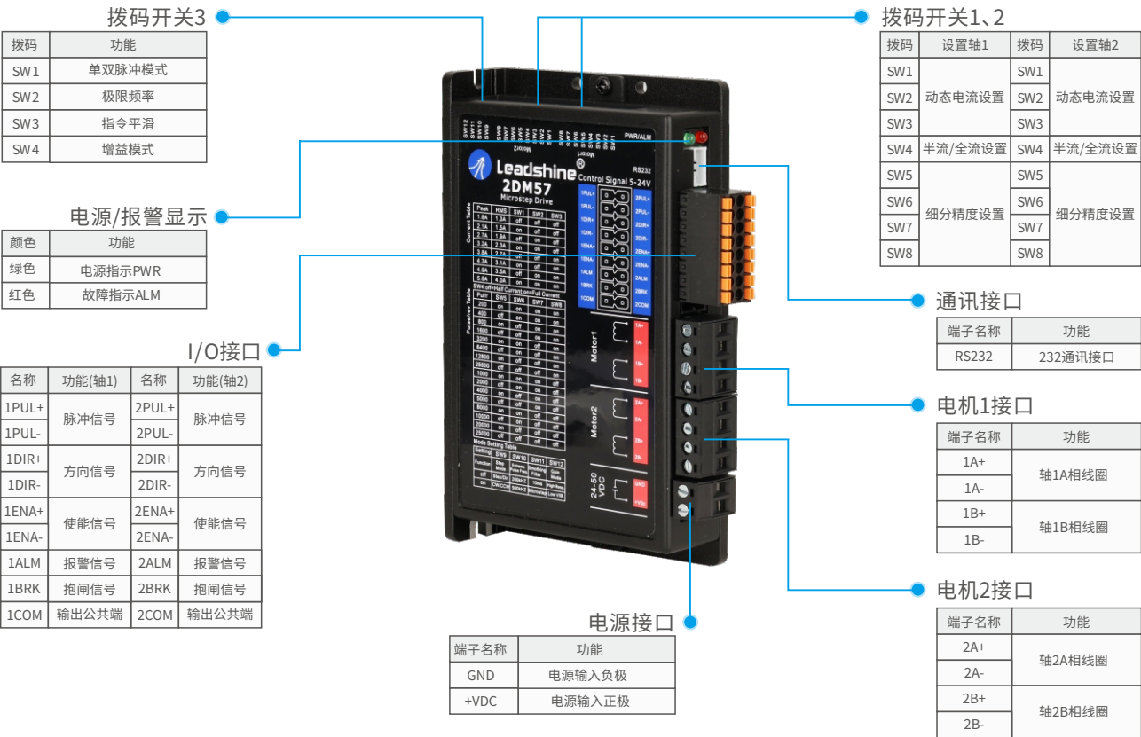
2DM57接口说明
