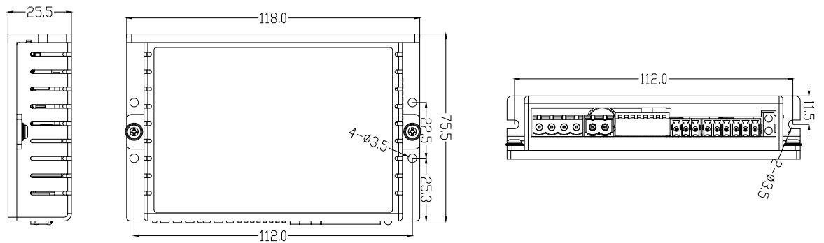
DM1-542安装尺寸图
