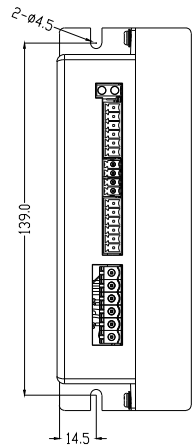
CL1-86C安装尺寸图
