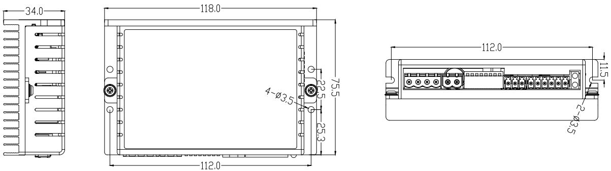
DM1-556、DM1-870安装尺寸图
