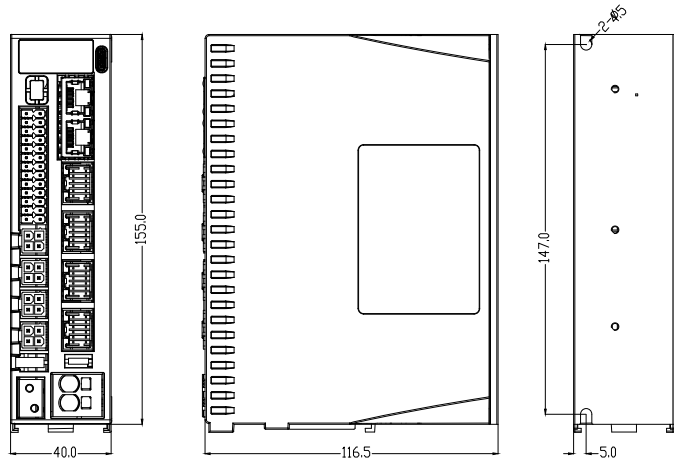
4CL3-EC503/507/808安装尺寸图
