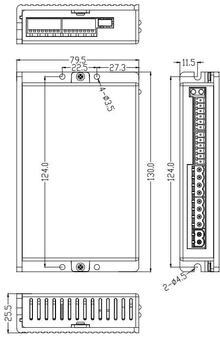
2DM86C 安装尺寸图
