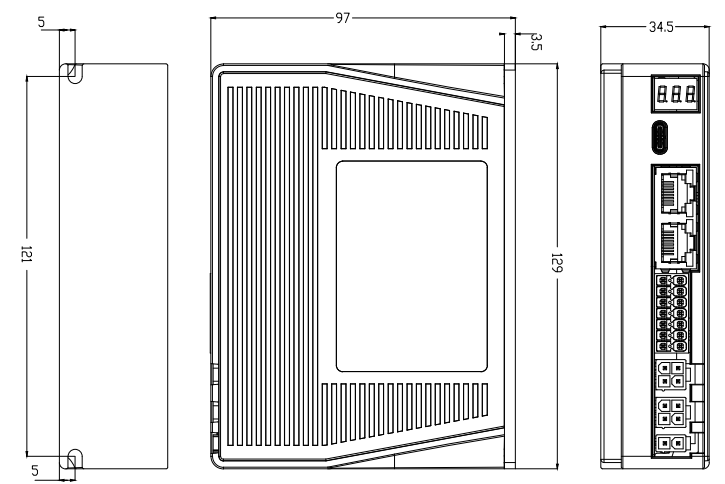
2DM3-EC556S安装尺寸图
