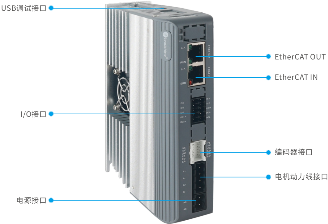
CL3B-EC808AC接口示意图
