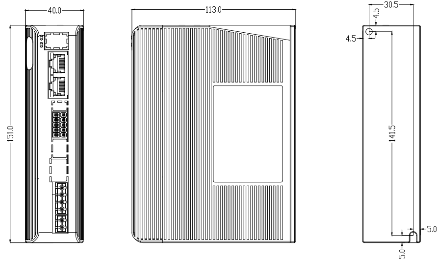
CL3B-EC808AC安装尺寸图
