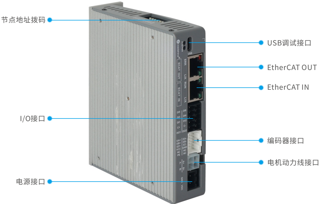
CL3B-EC503/507接口示意图
