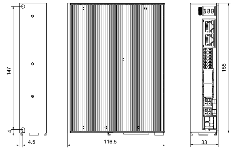
2DM3-EC882S安装尺寸图
