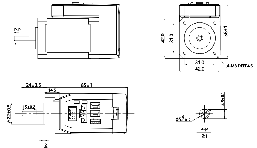
iCL42-RS08 (V2.0)
