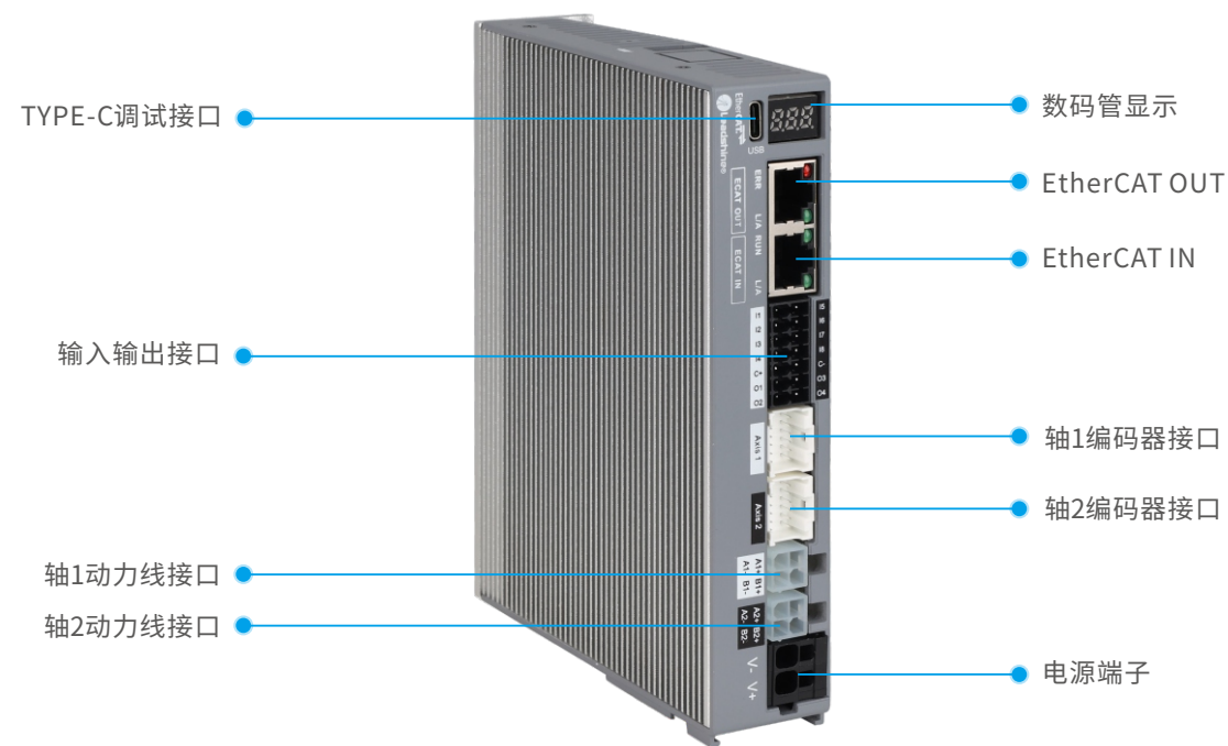
2CL3-EC808T接口示意图
