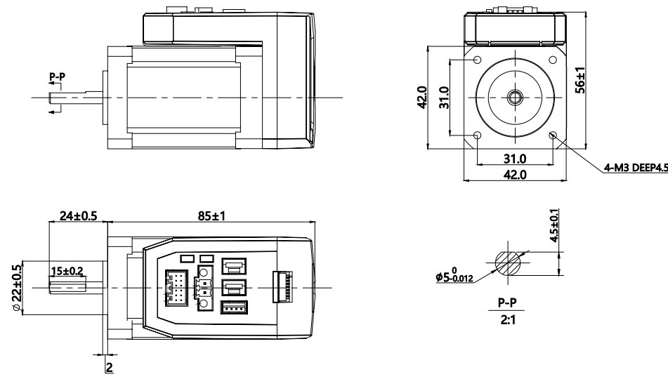
iDM42-RS08 (V2.0)
