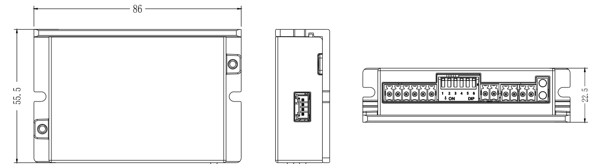
DM1-422C、DM1-432C安装尺寸图
