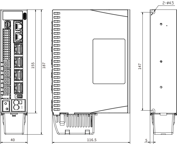
4CL3-ECS (带电池盒)
