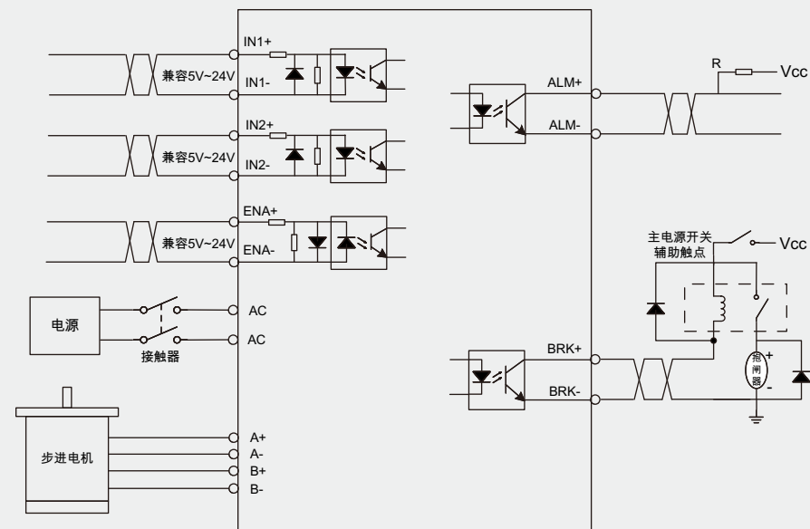
DM1-IO860C电气接线图
