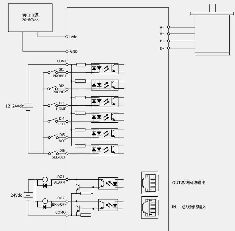
DM3B-EC522/542/556/570电气接线图
