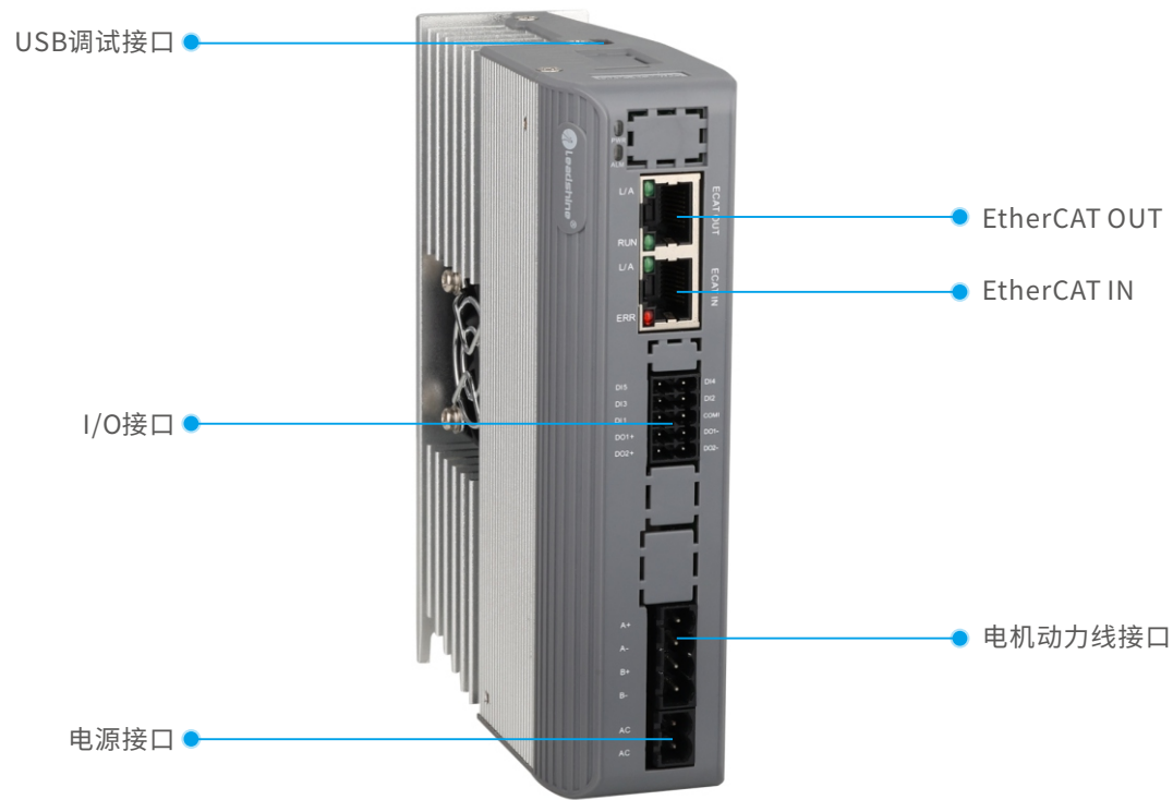
DM3B-EC882AC接口示意图
