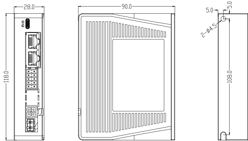
CL3B-EC503/507安装尺寸图
