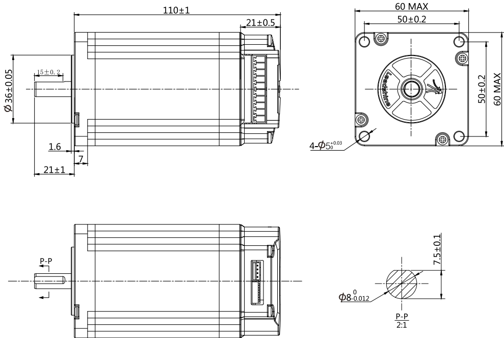
iCL60-30 (V2.0)
