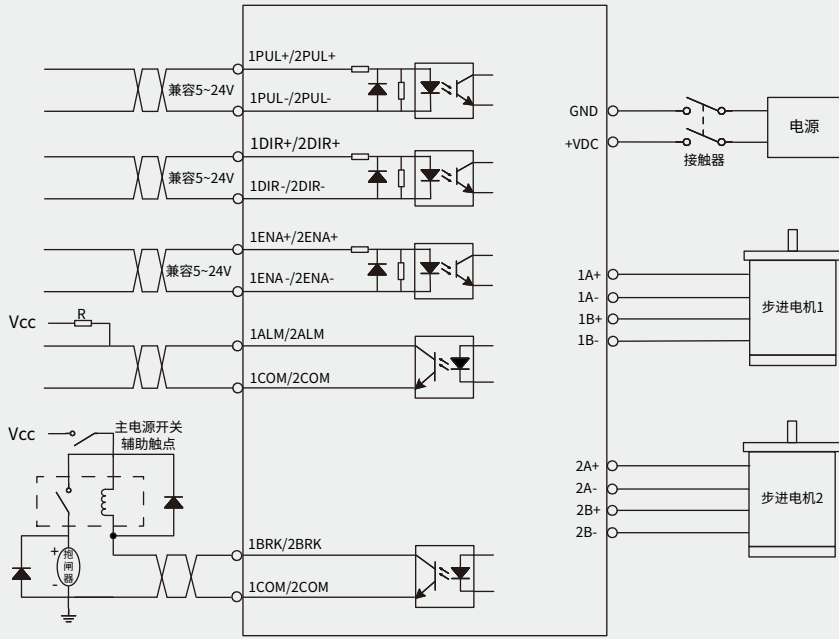
2DM57电气接线图
