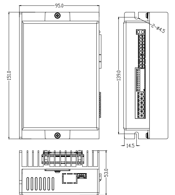
DM1-IO860C安装尺寸图
