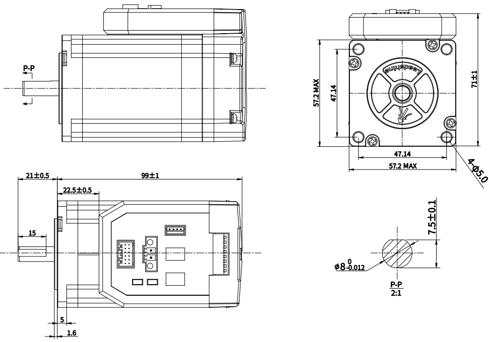
iDM57-RS23(V2.0)
