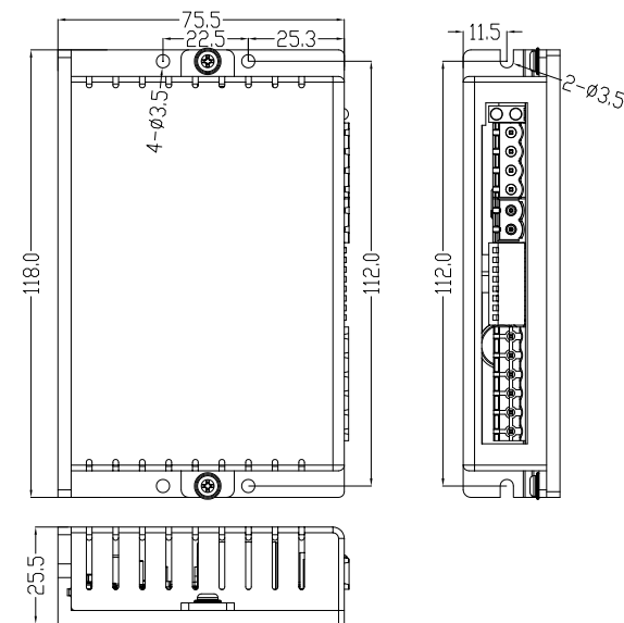
DM1-IO542C、DM1-IO556C安装尺寸图
