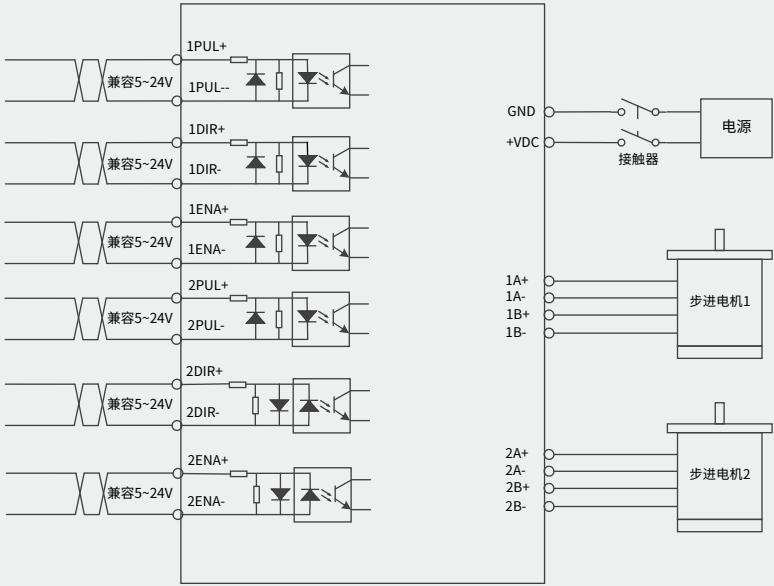
2DM42T、2DM57C、2DM86C电气接线图
