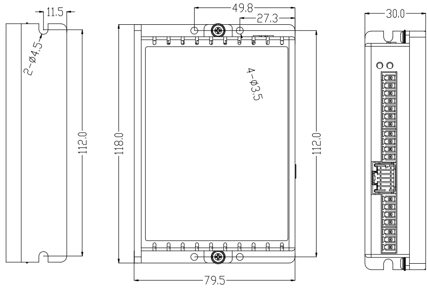
CL1-728安装尺寸图
