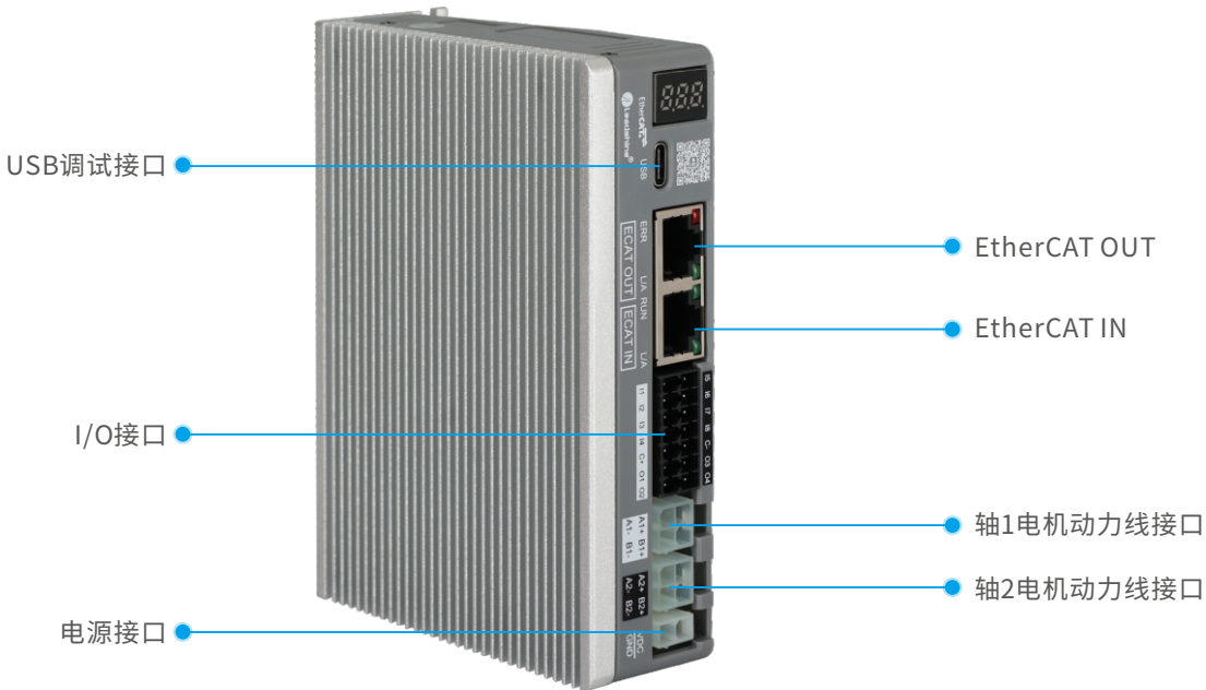
2DM3-EC432S/556S接口说明
