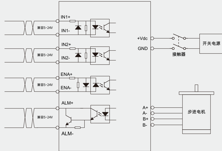
DM1-IO422C、DM1-IO442C、DM1-IO542C、DM1-IO556C电气接线图
