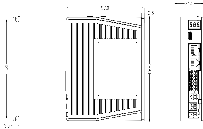
2CL3-EC403T/507T安装尺寸图
