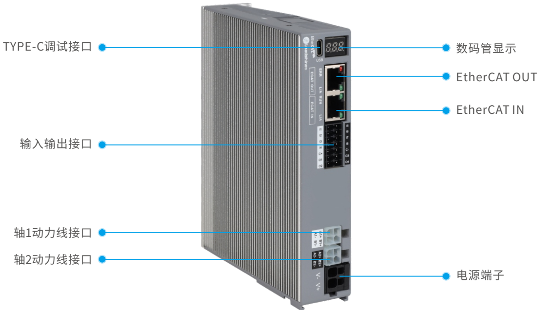
2DM3-EC882S接口说明
