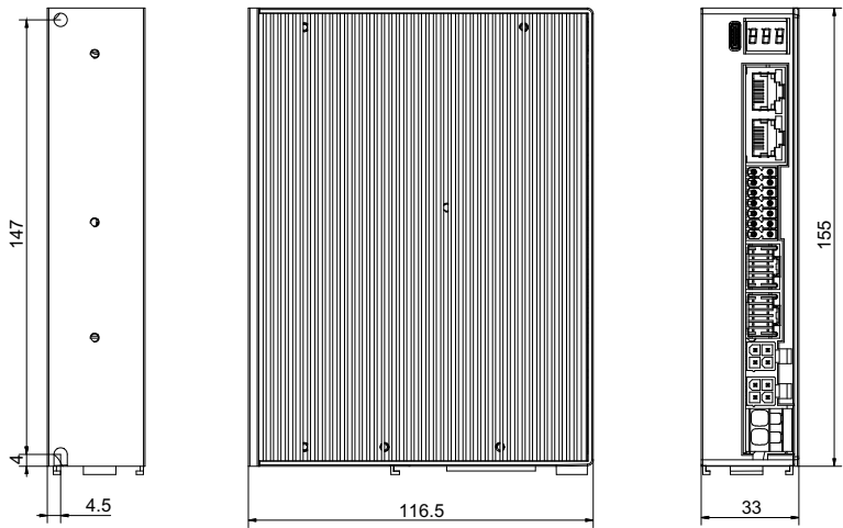
2CL3-EC808T安装尺寸图
