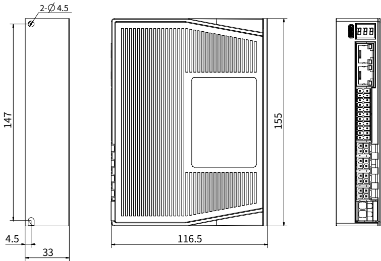
4DM3C-EC432/556 安装尺寸图
