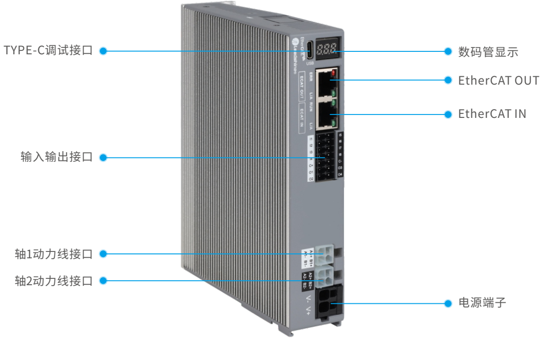
2DM3-EC882S接口说明
