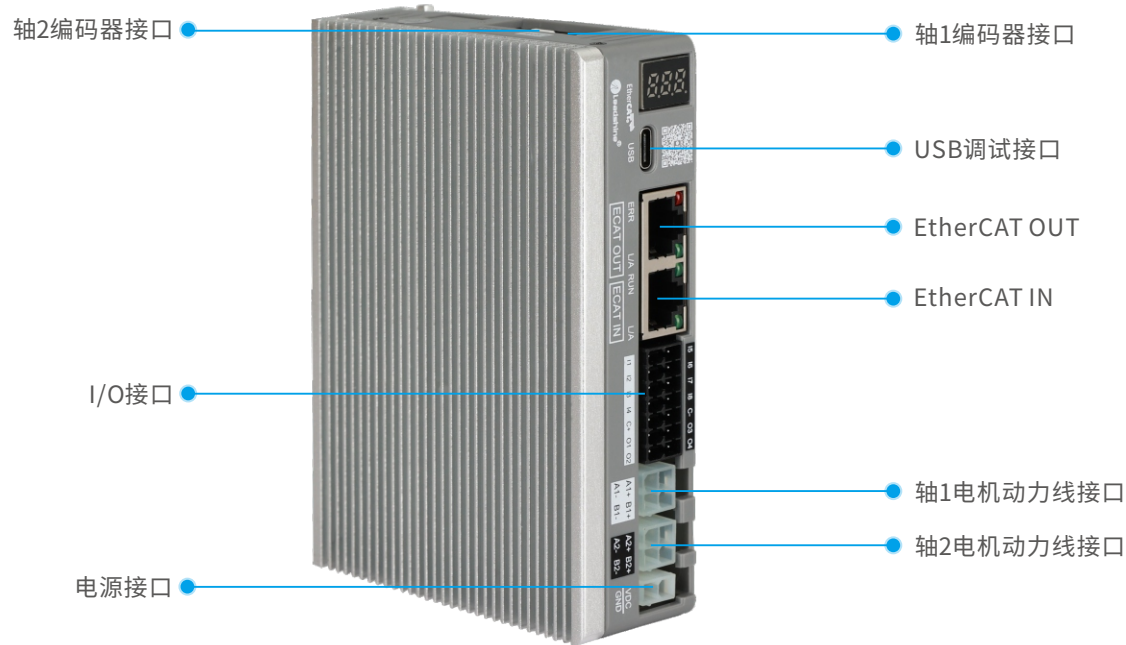
2CL3-EC507T/403T接口示意图
