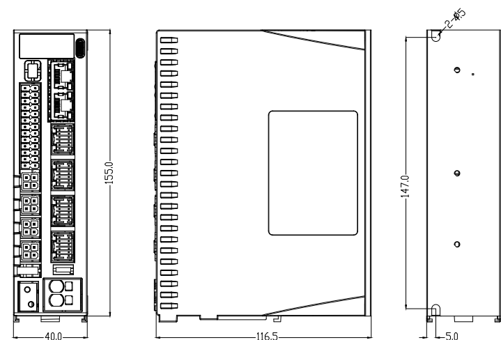
4CL3-EC503/507/808安装尺寸图
