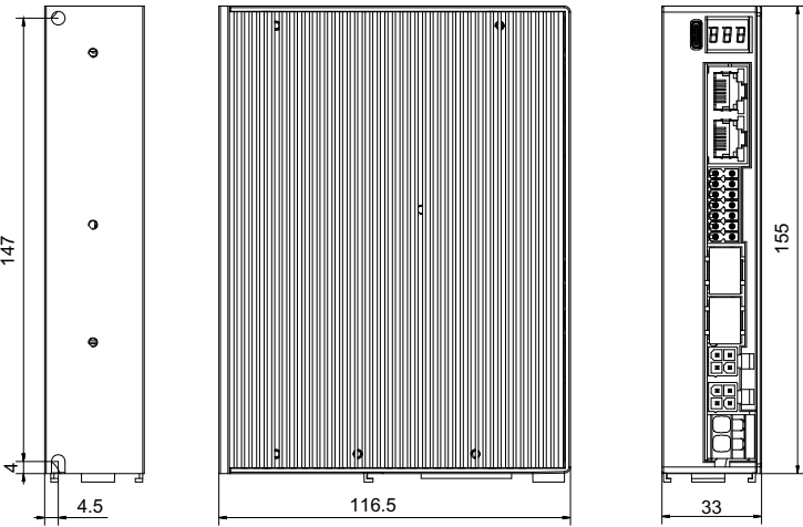
2DM3-EC882S安装尺寸图
