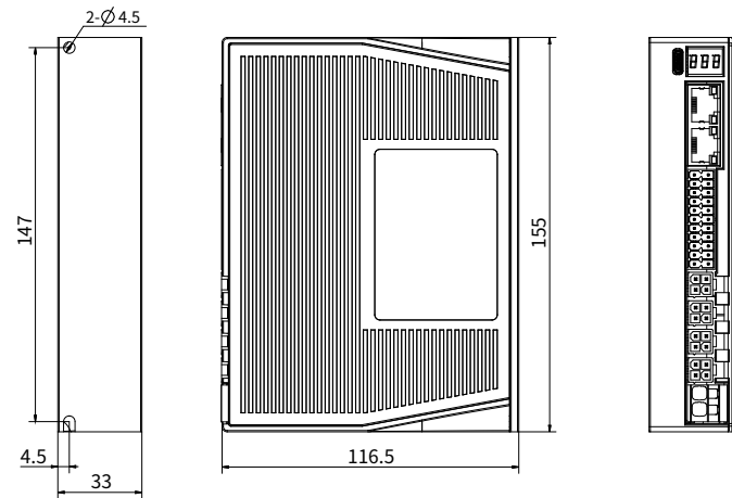
4DM3C-EC432/556 安装尺寸图
