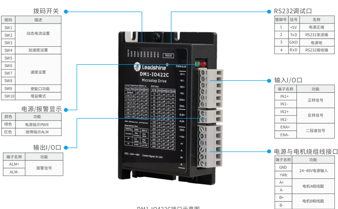
DM1-IO422C接口示意图
