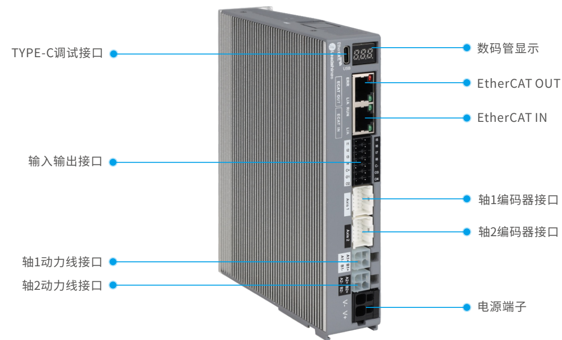
2CL3-EC808T接口示意图
