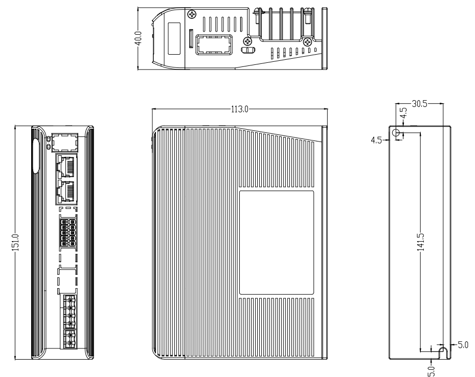
DM3B-EC882AC安装尺寸图
