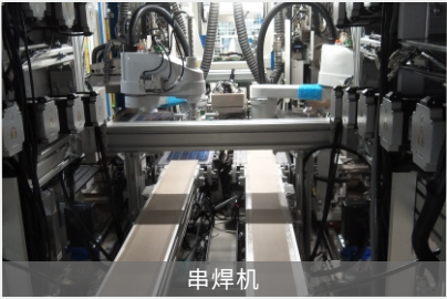
串焊机
