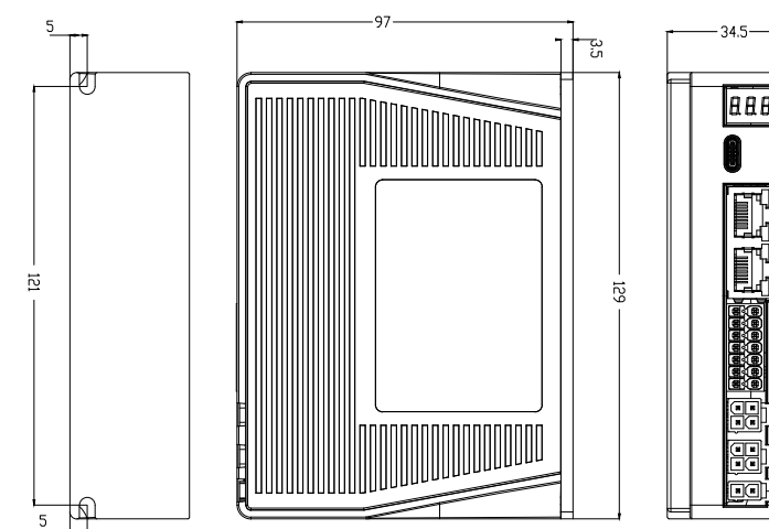
2DM3-EC556S安装尺寸图
