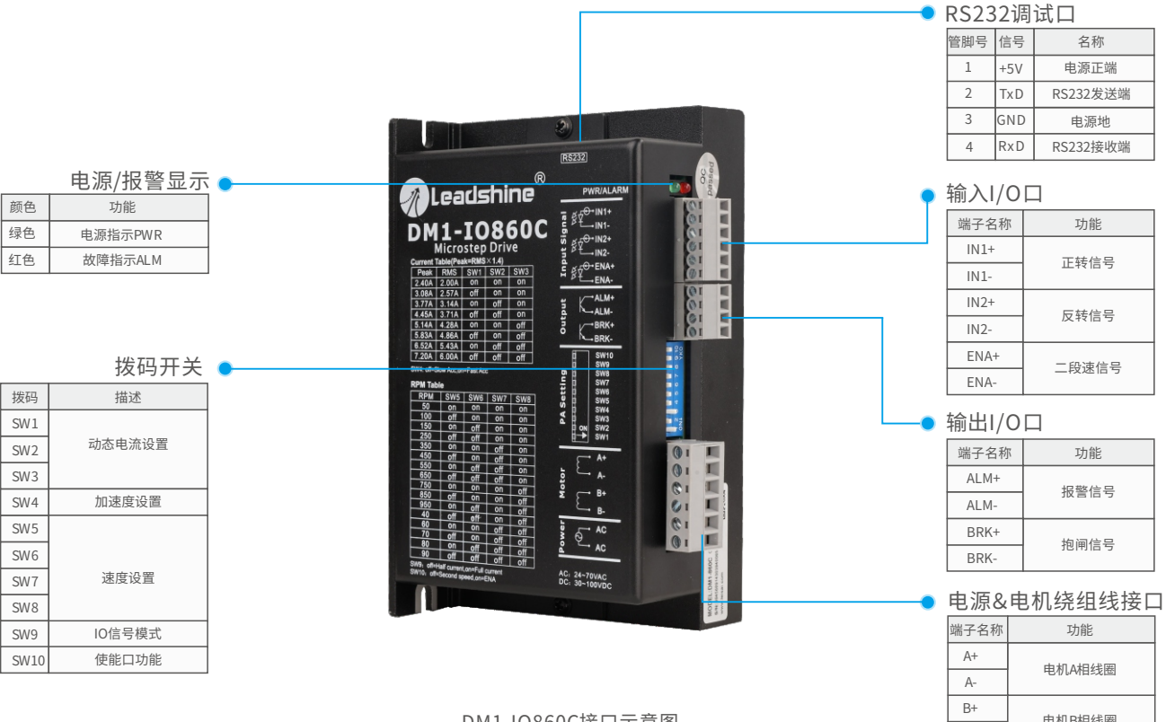
DM1-IO860C接口示意图
