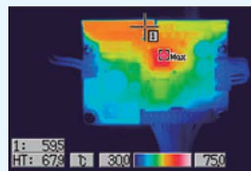
相同运行条件下测试记录的电机温度分布图
