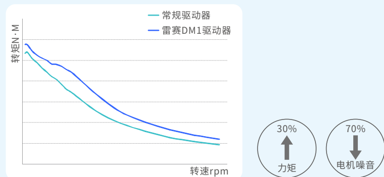
DM1系列驱动器与传统驱动器匹配同一电机(同一条件)的转矩图
