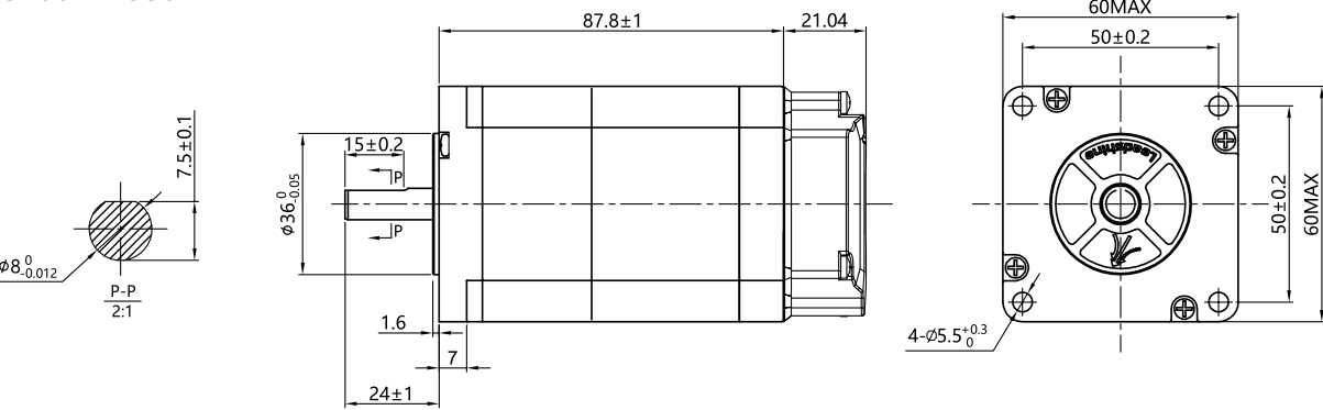
iCL60A-RS30
