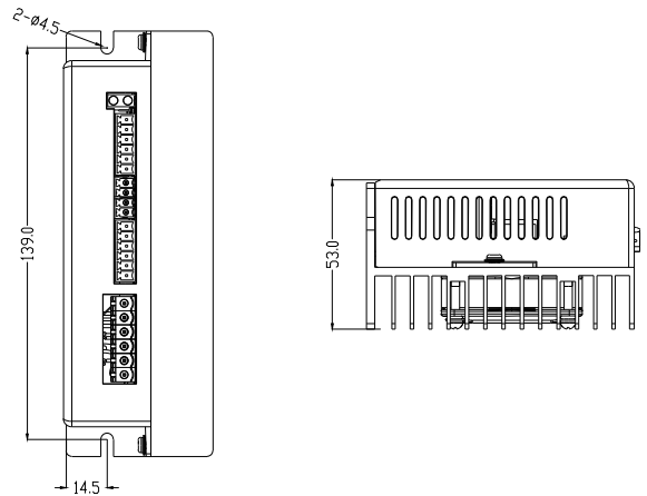
CL1-86C安装尺寸图
