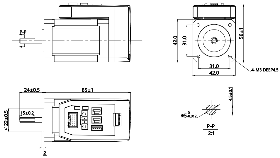
iDM42-RS08 (V2.0)
