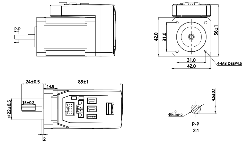
iCL42-RS08 (V2.0)
