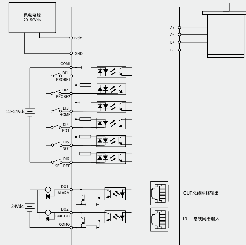
DM3B-EC522/542/556/570电气接线图
