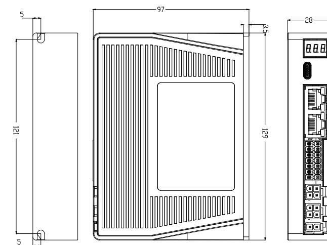
2DM3-EC432S安装尺寸图
