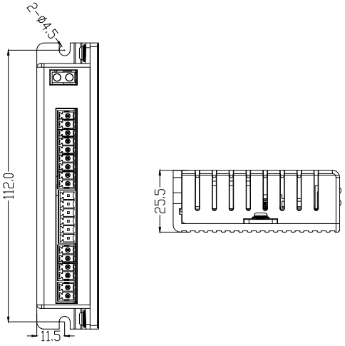
CL1-42C/57C安装尺寸图
