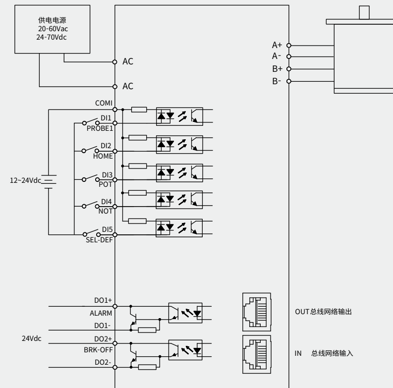
DM3B-EC882AC电气接线图
