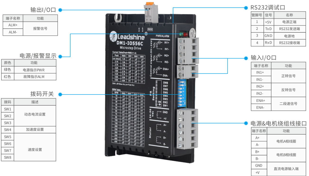
DM1-IO442C、DM1-IO542C、DM1-IO556C接口示意图
