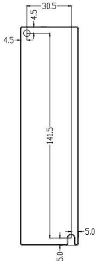
图 2-1 CL3B-EC808AC 安装尺寸图 (单位: mm)
