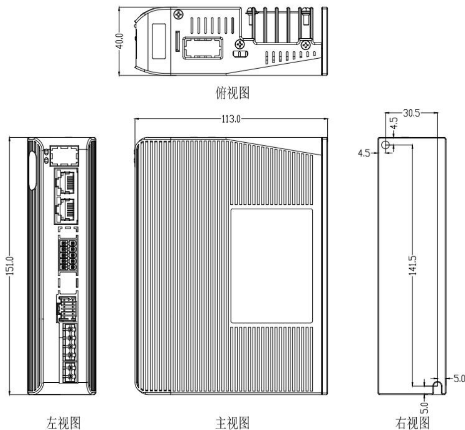
图 2-1 CL3B-EC808AC 安装尺寸图(单位: mm)
